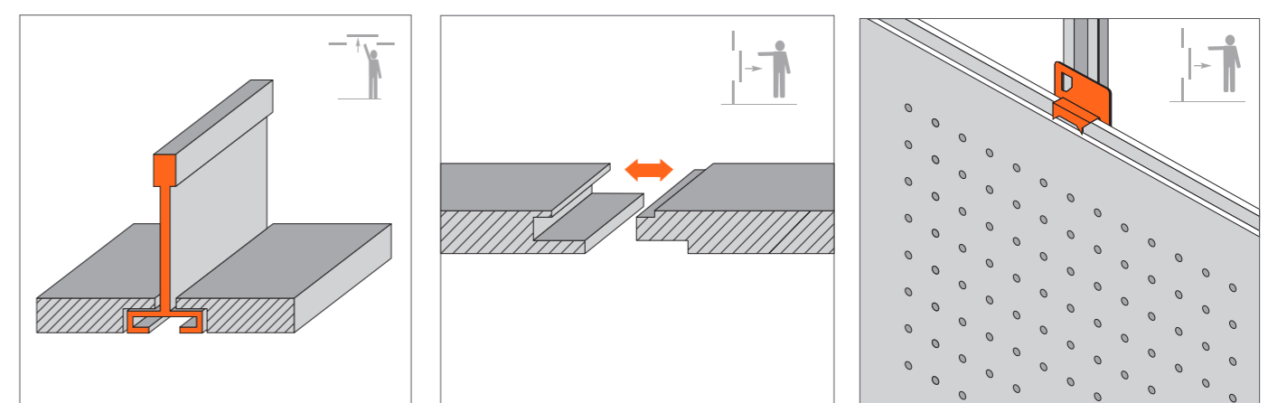
PERFIL FINELINE T-15 FINELINE FORM T-15
