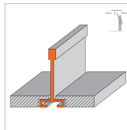
PERFIL FINELINE T-15 FINELINE FORM T-15
